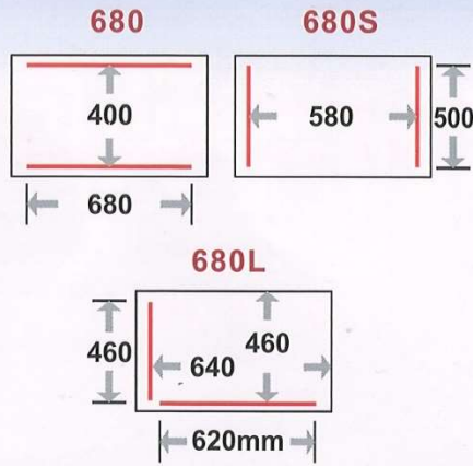
封口座位置標示圖
