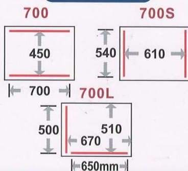
封口座位置標示圖
