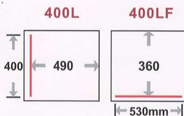
封口座位置標示圖
