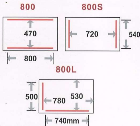
封口座位置標示圖
